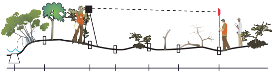
Figura 20. Nivelación con un instrumento de estación total. Símbolos cortesía de la integración y la red de aplicaciones ( ian.umces.edu/symbols/ ).
