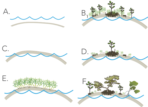
Figura 28. Proceso de construcción de un centro de nucleación: A) Un suelo sobre inundado, B) Se realiza la elevación del suelo sobre el nivel del agua, C) El establecimiento de las especies pioneras, D) Llegan los primeros propágulos de manglar, E) Se establecen las plántulas de manglar, disminuye la vegetación pionera y, por último, F) Se hace el reclutamiento de diferentes especies de manglar. Símbolos cortesía de la integración y la red de aplicaciones (ian.umces.edu/symbols/).
