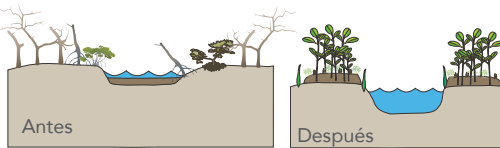
Figura 27. Imagen que representa una zona, antes y después de la construcción de un centro de nucleación, como parte de las acciones de restauración. Símbolos cortesía de la integración y la red de aplicaciones ( ian.umces.edu/symbols/ ).
