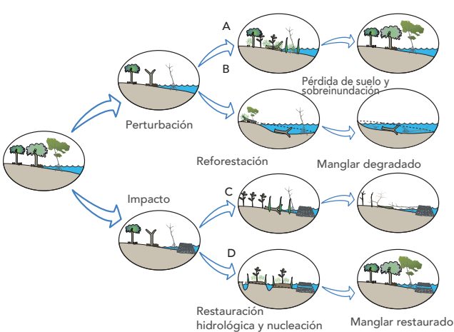
Figura 11. Las perturbaciones naturales (A y B) y los impactos por el cambio del uso del suelo (B y C), alteran los patrones de la hidrología y dañan la vegetación. En el caso A, por regeneración natural el manglar puede recuperarse. Sin embargo, cuando esto no ocurre el manglar continúa su degradación, hay pérdida de suelo y sobre inundación (caso B). En el caso C, cuando hay alguna modificación física en el terreno, el hidroperíodo y la vegetación son afectados; y cuando se emplea la reforestación, los resultados no son los esperados (caso C). Por último, en el caso D, las acciones de restauración hidrológica y la regeneración inducida por nucleación, tienen mejores resultados en la recuperación del manglar, en un menor tiempo. Tomado y modificado a partir de Lewis et al., 2015. Símbolos cortesía de la integración y la red de aplicaciones (ian.umces.edu/symbols/).
