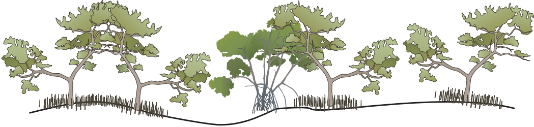
Figura 8. Distribución típica de los manglares tipo cuenca en Panamá. Símbolos cortesía de la integración y la red de aplicaciones ( ian.umces.edu/symbols/ ).
